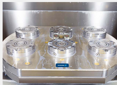
Die VERO-S Spannstation ist eine Präzisionschnittstelle zum Maschinentisch und ermöglicht das schnelle Rüsten jeglicher Spannelemente.
